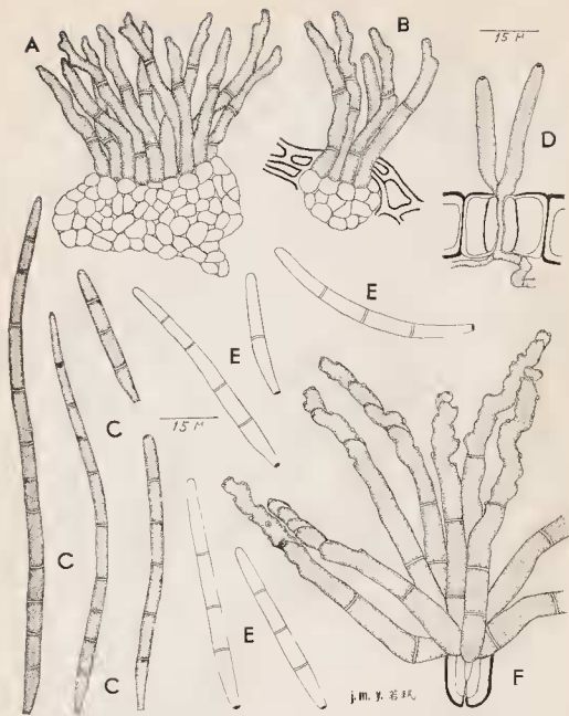
Fig. 4. Cercospora melochiae P. Henn. (A-C): A, Fascicule de conidiophores dense et stroma; B, Fascicule maigre et stroma rudimentaire; C, Conidies. Cercospora sorghi Ed. et Ev. (D-F): D, Conidiophores jeunes; E, Conidies; F, Fascicule de conidiophores âgés.
